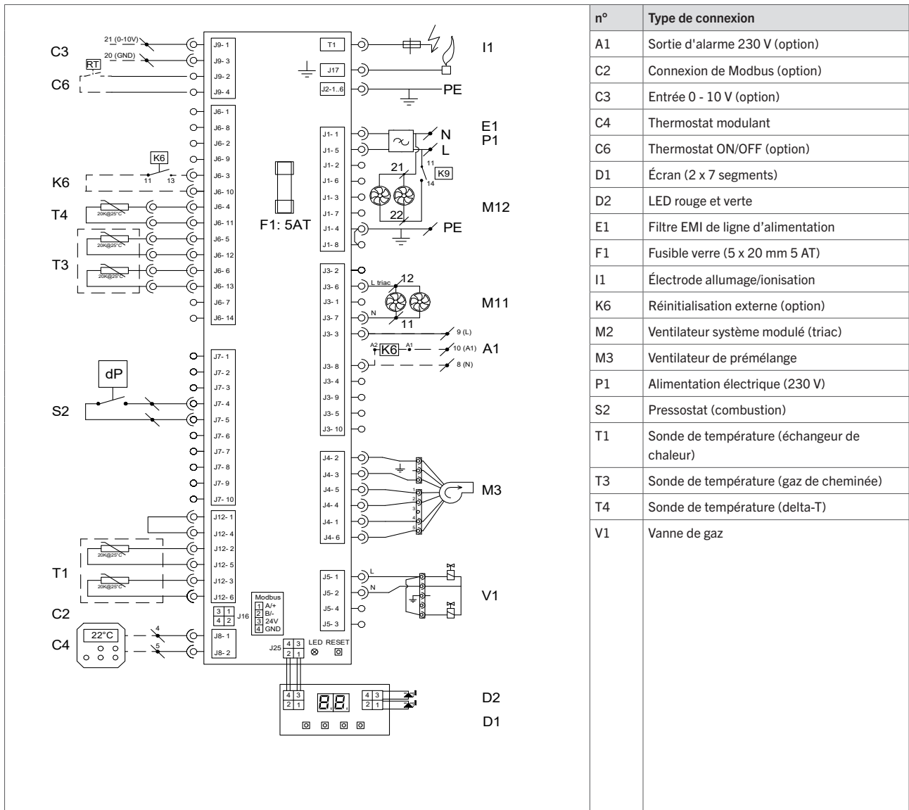
Figure 31 - Schéma de câblage TRX+78 - TRX+117 AC
