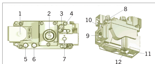
Figure 23 - Composants majeurs de la vanne de gaz TRX+78 - TRX+117
