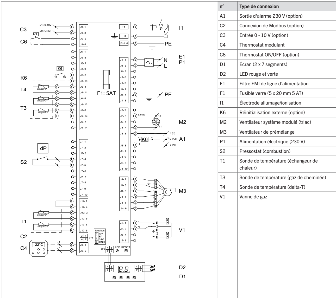
Figure 27 - Schéma de câblage TRX+14 - TRX+65 AC
