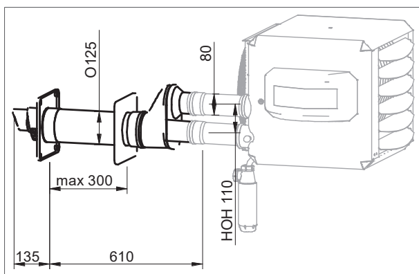
Figure 17 - Terminal horizontal des gaz de cheminée TRX+14 - TRX+117
