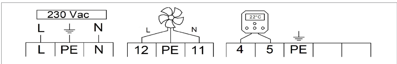
Figure 28 - Principales connexions d'installation TRX+14 - TRX+65 AC
