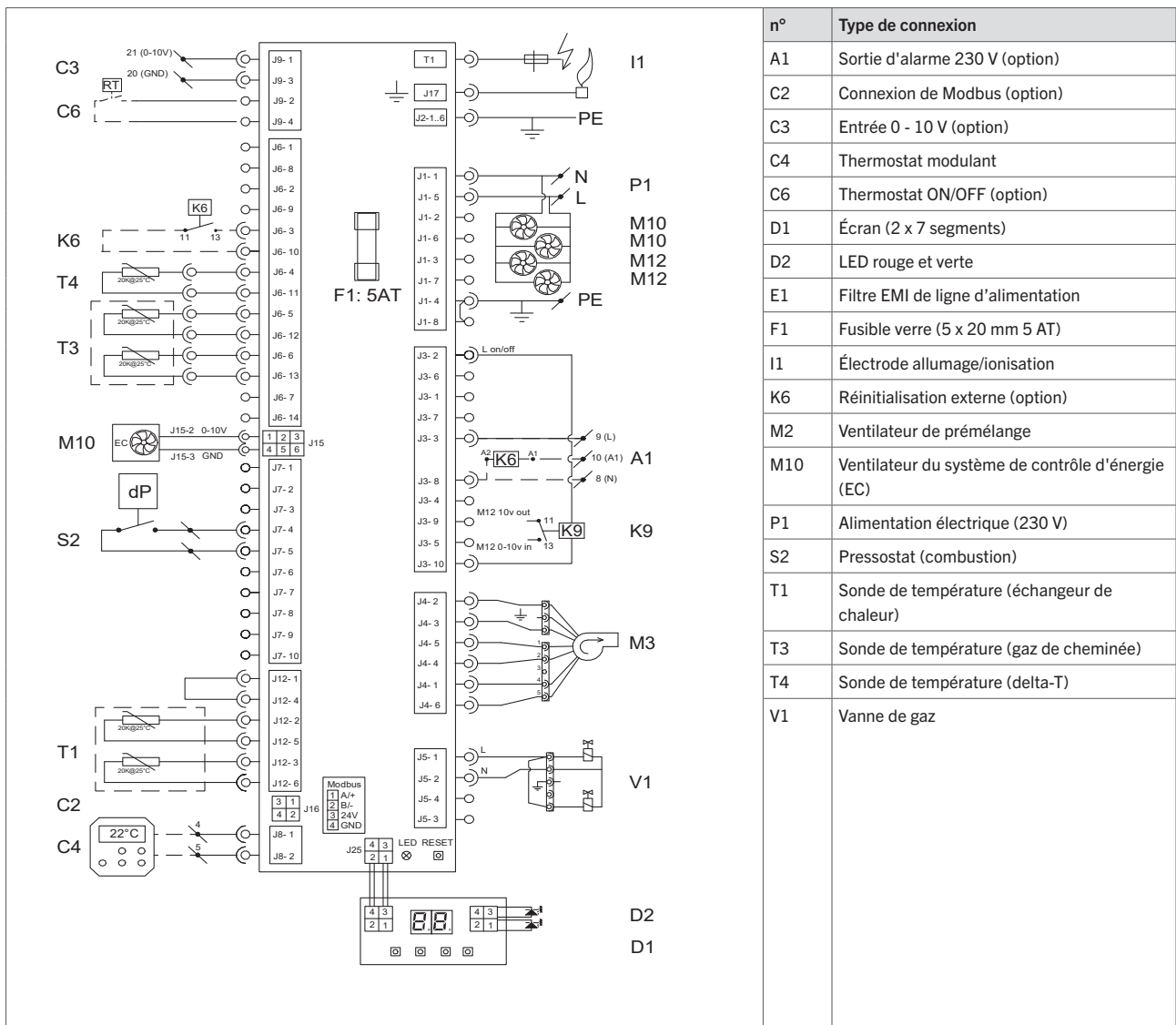
Figure 33 - Schéma de câblage TRX+78 - TRX+117 EC
